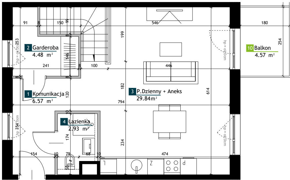
POZIOM GÓRNY
