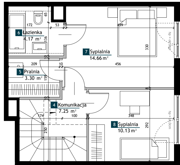
POZIOM DOLNY
