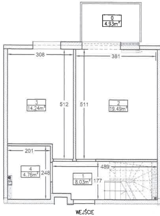
Szkic lokalizacji rzut 3 piętra
